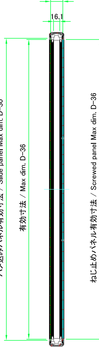
B-B (1 : 5.5)
